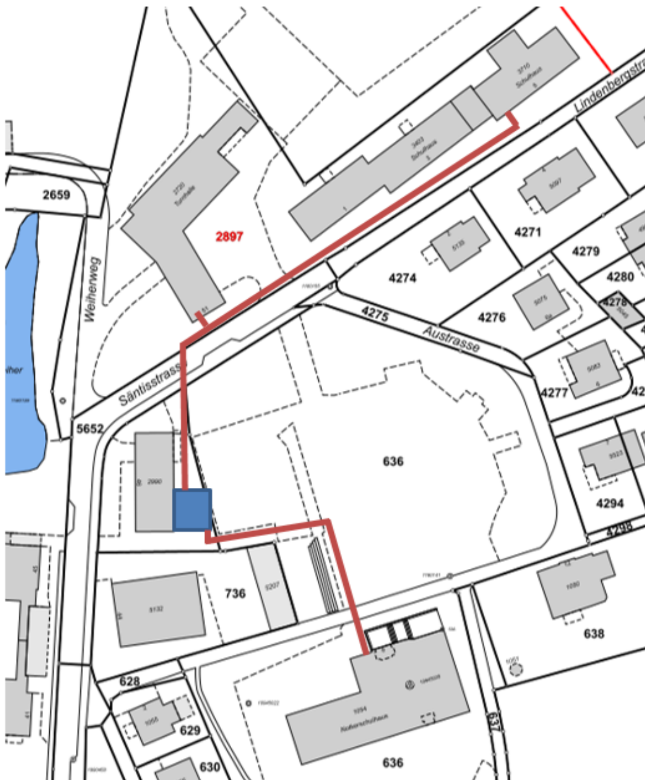
Situation Wärmeverbund mit Zentrale «Schulhaus am Weiher» (Machbarkeit 7.5)
