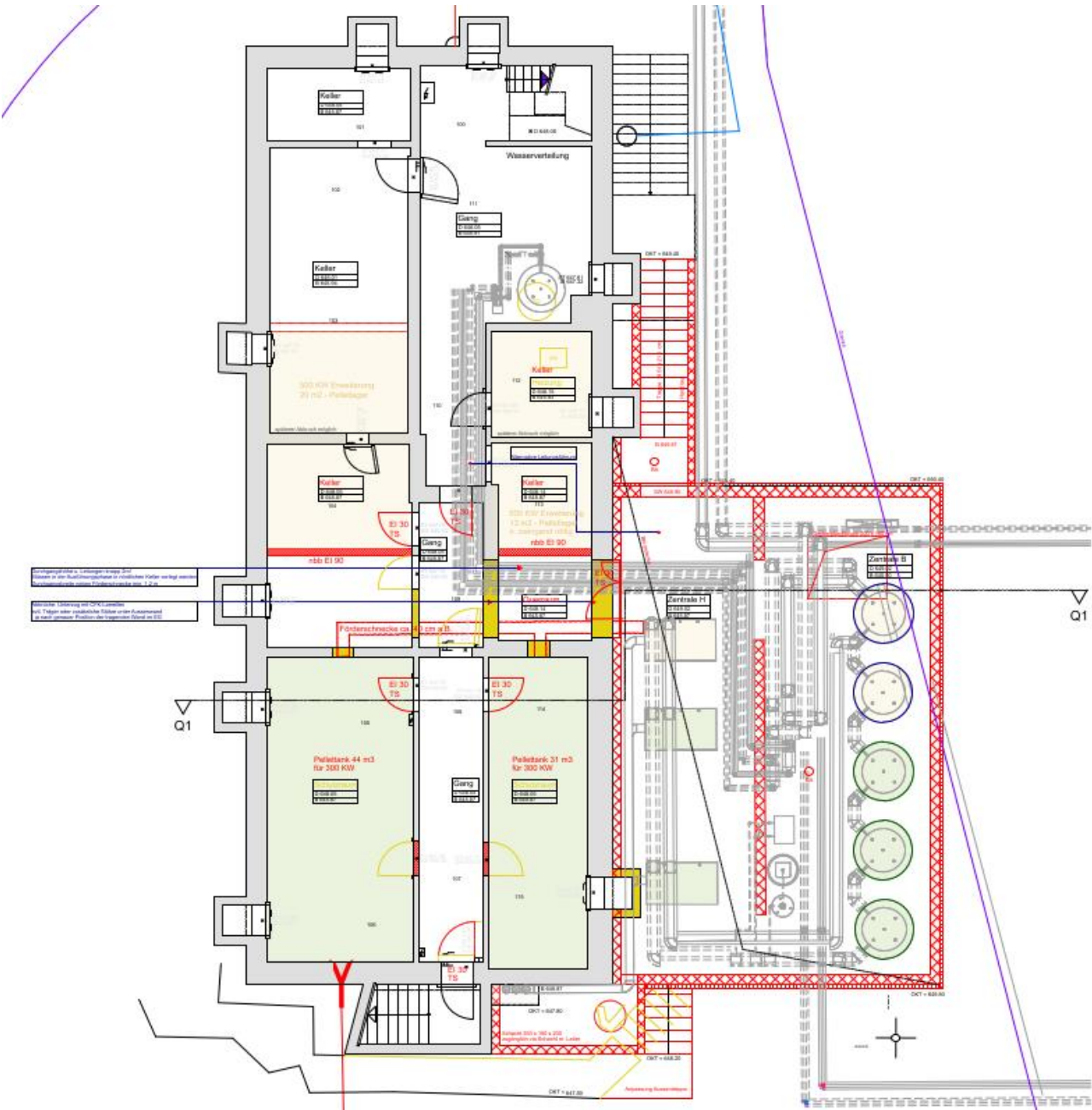
Grundriss Wärmeerzeugungszentrale «Schulhaus am Weiher»
