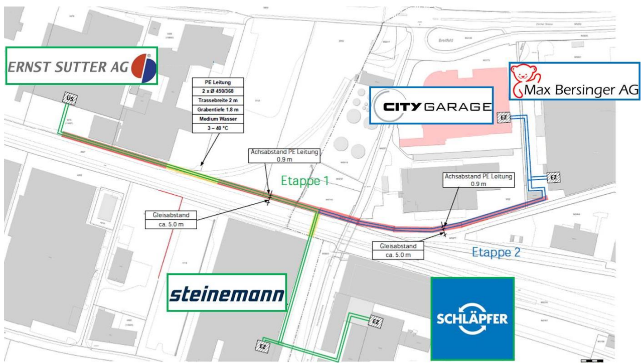
Abbildung 1: Ausbauetappen 1 und 2 (Initialcluster)
